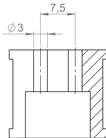
SCHNITT A-A
